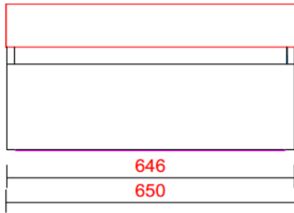
WASTAFEL VOOR-AANZICHT
