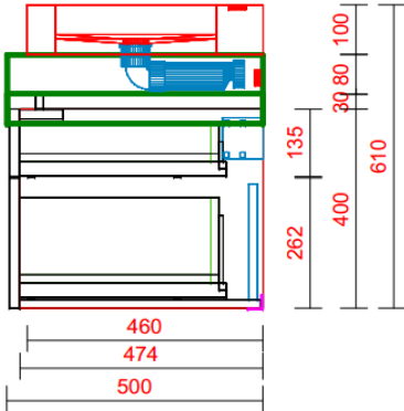
WASTAFEL ZIJ-AANZICHT
