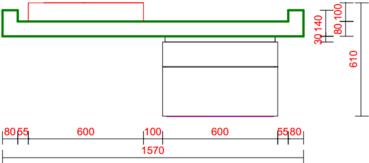
WASTAFEL VOOR-AANZICHT
