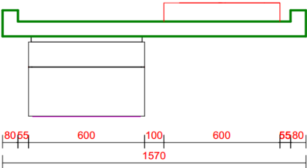
WASTAFEL VOOR-AANZICHT
