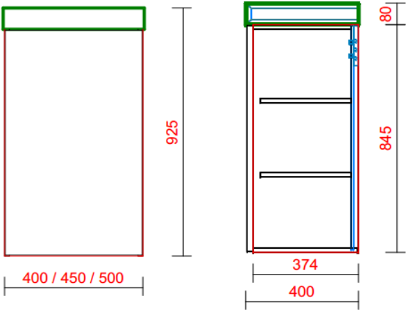
VOOR-AANZICHT KOLOMKAST MET ELEMENT ZIJ-AANZICHT KOLOMKAST MET ELEMENT
