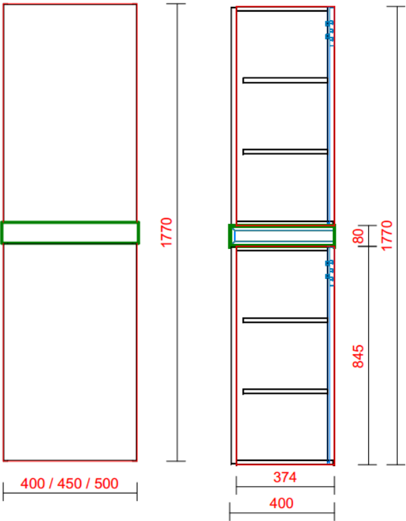
VOOR-AANZICHT KOLOMKAST MET ELEMENT ZIJ-AANZICHT KOLOMKAST MET ELEMENT
