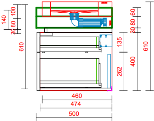
WASTAFEL ZIJ-AANZICHT
