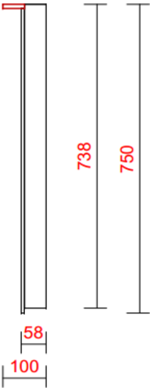
ZIJ-AANZICHT SPIEGEL
