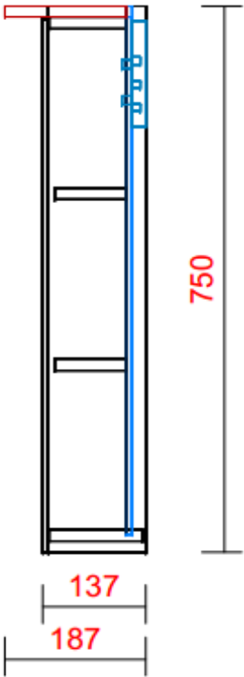
ZIJ-AANZICHT SPIEGELKAST
