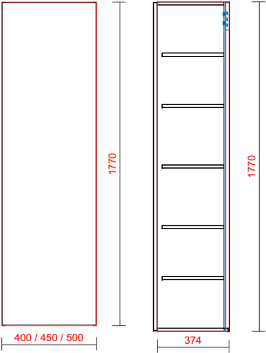
VOOR-AANZICHT KOLOMKAST ZIJ-AANZICHT KOLOMKAST
