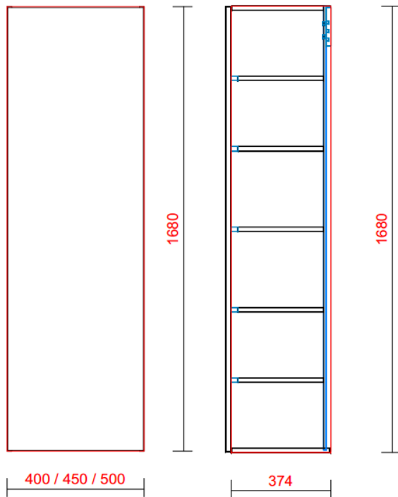
VOOR-AANZICHT KOLOMKAST
