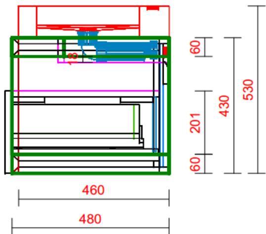
ZIJ-AANZICHT WASTAFEL
