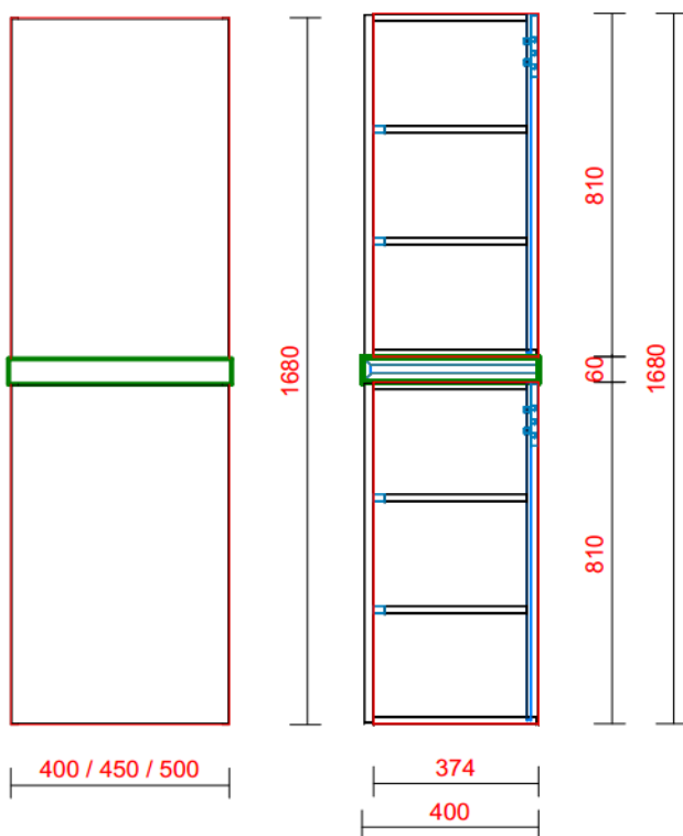
VOOR-AANZICHT KOLOMKAST MET ELEMENT
