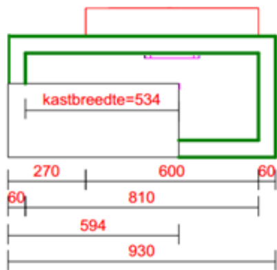
WASTAFEL VOOR-AANZICHT LINKS
