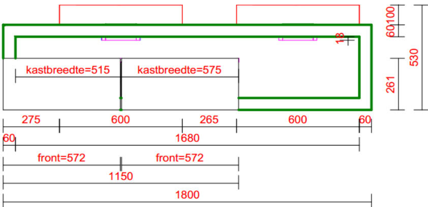
WASTAFEL VOOR-AANZICHT LINKS
