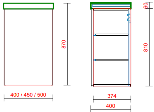
VOOR-AANZICHT KOLOMKAST MET ELEMENT
