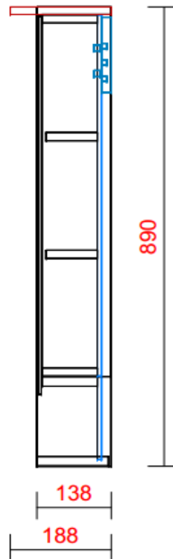
ZIJ-AANZICHT SPIEGELKAST MET REGAAL
